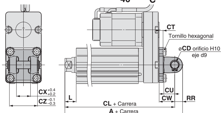
Fijación oscilante hembra: LEY32 \square\square \begin{matrix} 25 \\ 40 \\ A \\ B \\ C \end{matrix} - \square\square\square D
