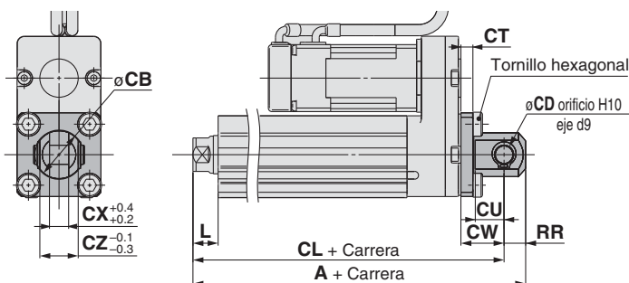
Fijación oscilante hembra: LEY32 \square\square \begin{matrix} 25 \\ 40 \\ A \\ B \\ C \end{matrix} - \square\square\square D
