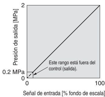
Fig. 1. Gráfico de características de entrada/salida
