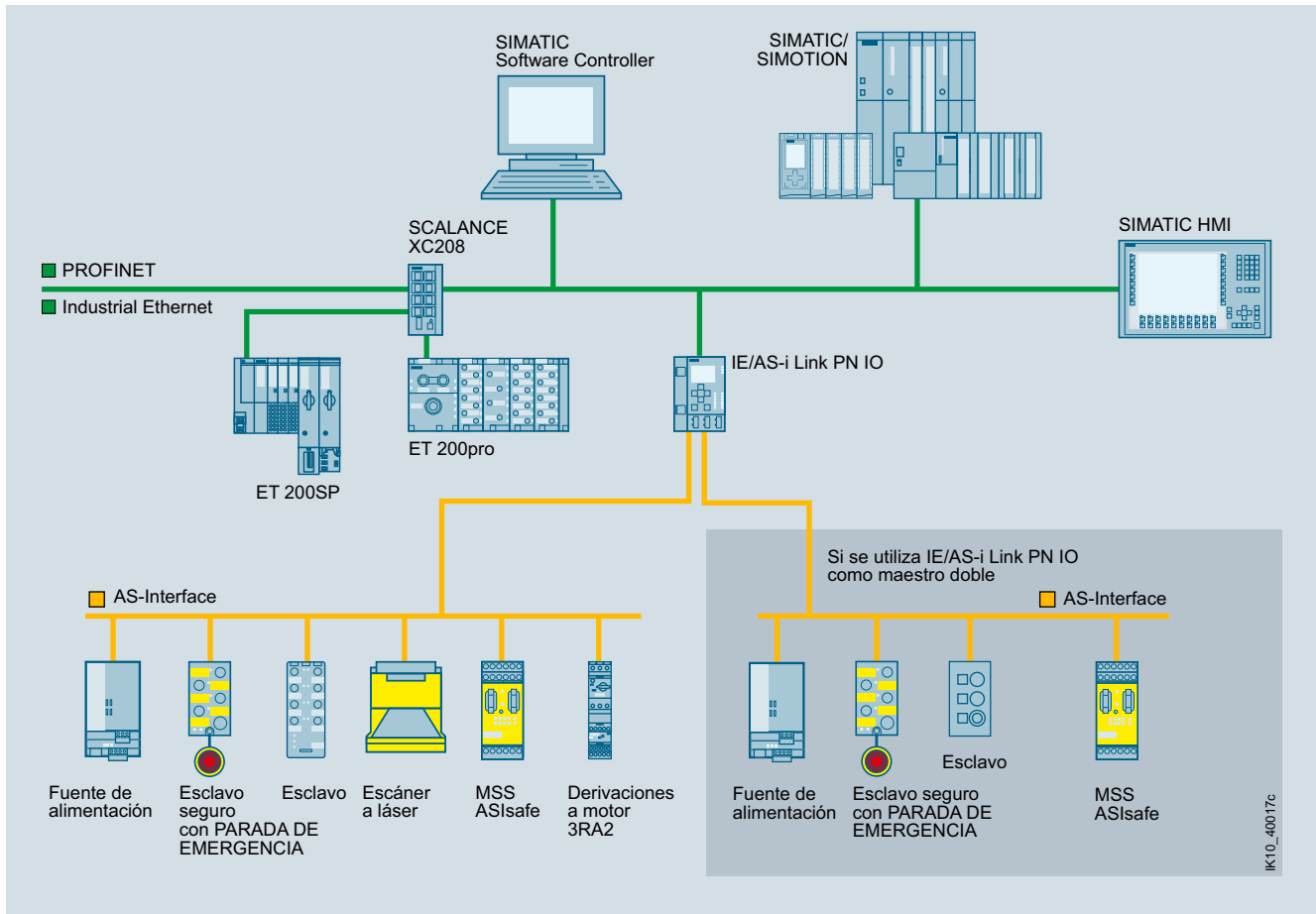
Conexión de AS-Interface a PROFINET vía IE/AS-i Link PN IO como maestro simple y doble
