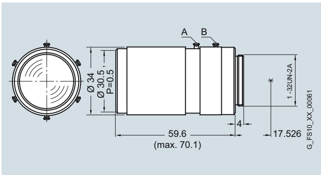
Lens 6GF9001-1BK01
