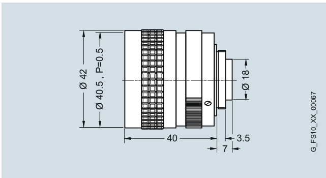
Lens 6GF9001-1BE01
