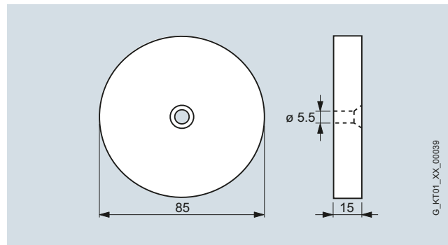
MDS D139 transponder
