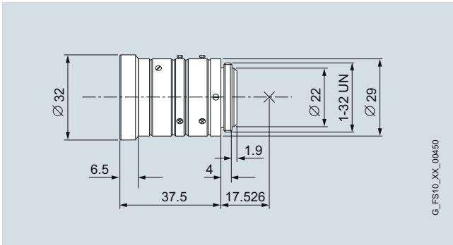
Lens 6GF9001-1BB01
