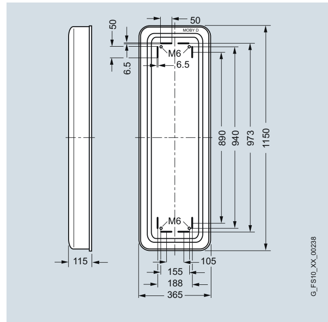
ANT D10 antenna
