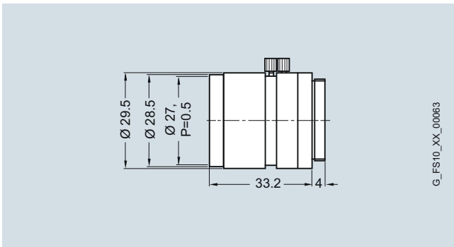
Lens 6GF9001-1BF01
