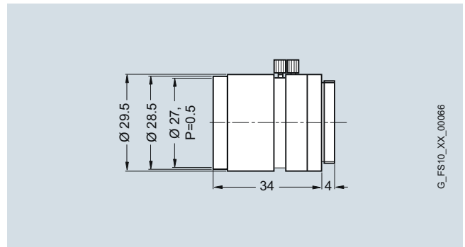
Lens 6GF9001-1BJ01
