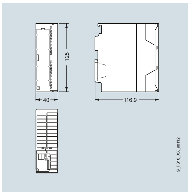
ASM 475 communication module
