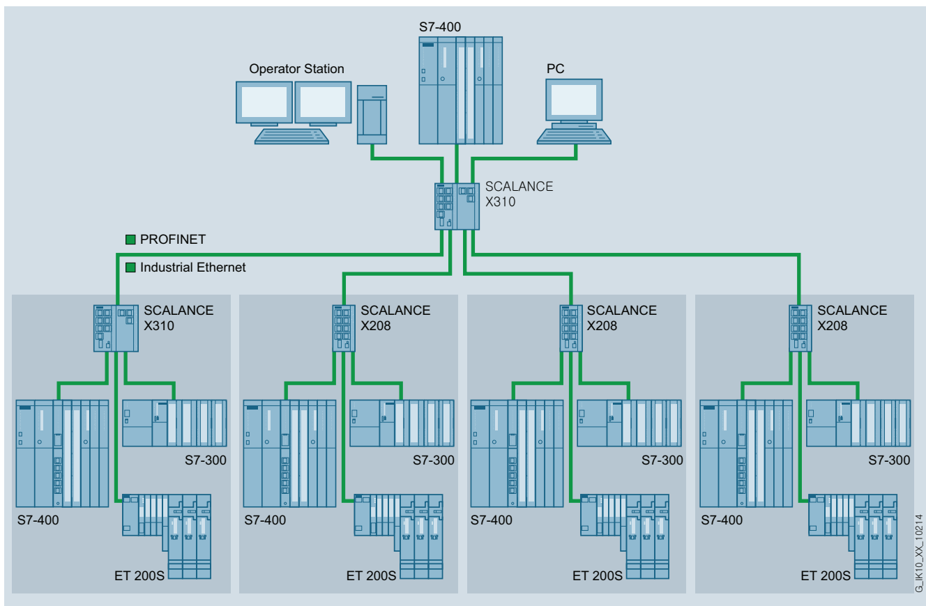
Topología eléctrica en estrella con SCALANCE X310
