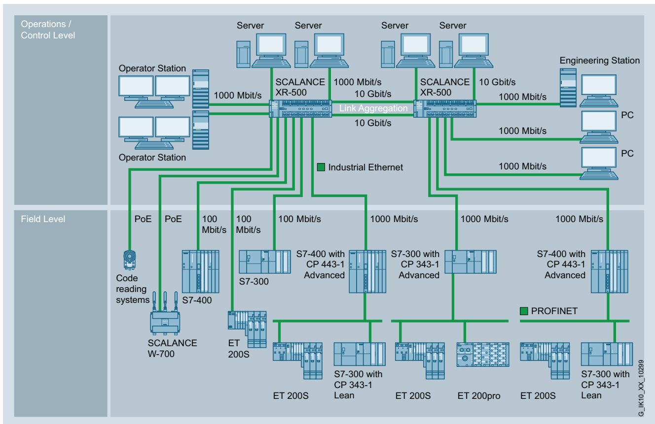
Aumento del ancho de banda de transferencia mediante Link Aggregation
