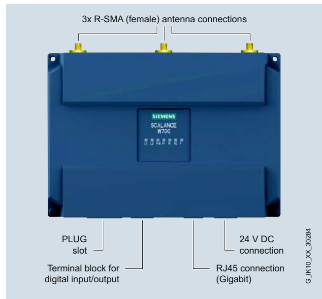
Diseño mecánico e interfaces de los módulos cliente SCALANCE W748-1 RJ45
