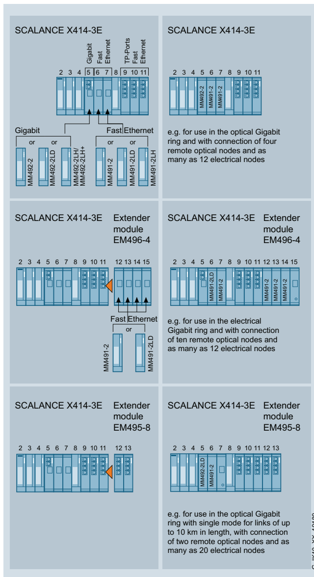
Posibilidades de aplicación de los módulos de medio y de extensión con SCALANCE X414-3E
