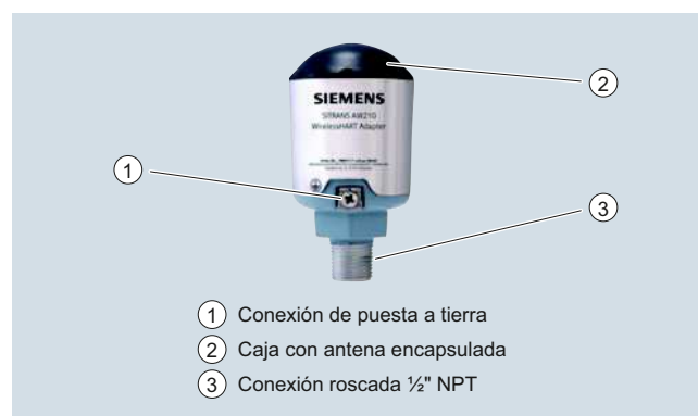
Adaptador Wireless HART SITRANS AW210, estructura
