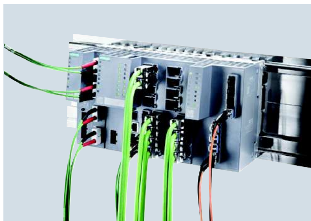
Cable de conexión FO Cord SC/SC entre XC100-4OBR y SCALANCE X320-3LD
