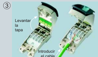
Conexión del cable
