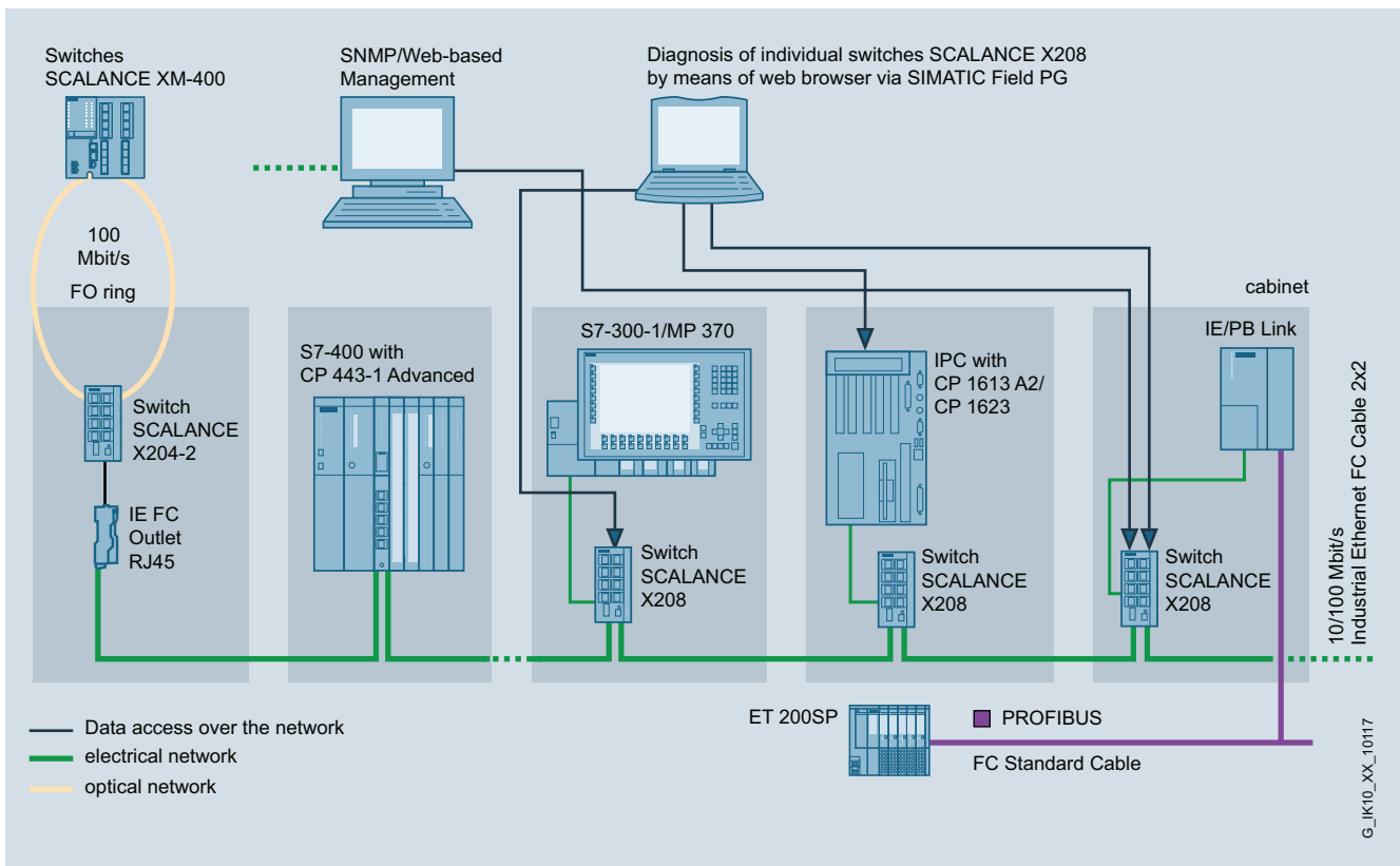
Acceso al diagnóstico vía SNMP y navegador web con SCALANCE X208
