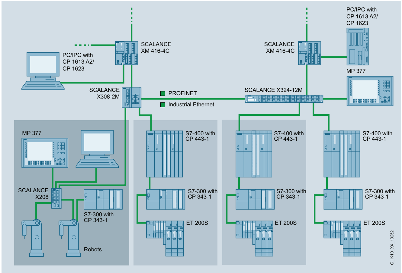
Comutación en la capa 3 de alto rendimiento junto con un encaminamiento redundante (VRRP)
