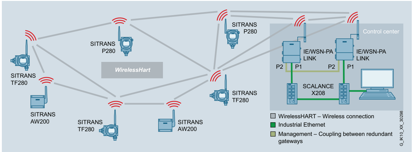
Red WirelessHART funcionando con pasarela redundante
