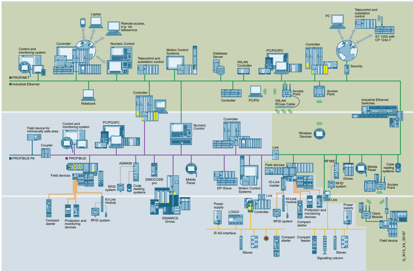
Industrial Ethernet en el entorno de comunicación
