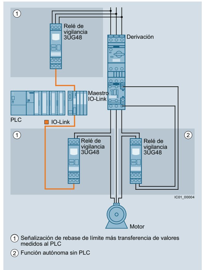
Relés de vigilancia para IO-Link
