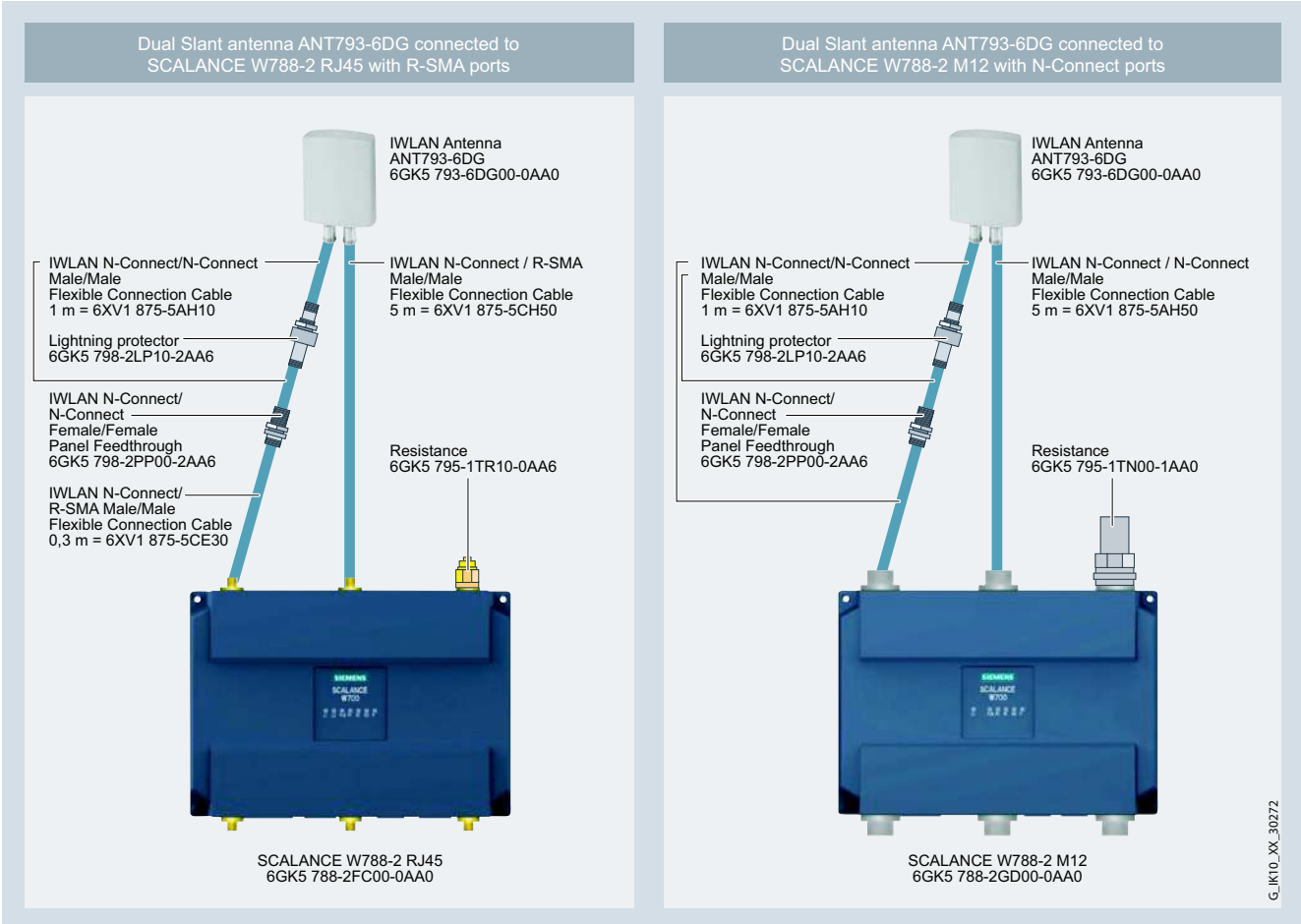
Puntos de acceso SCALANCE W788-1 RJ45 con antena Dual Slant y SCALANCE W788-1 M12 con conexión N-Connect
