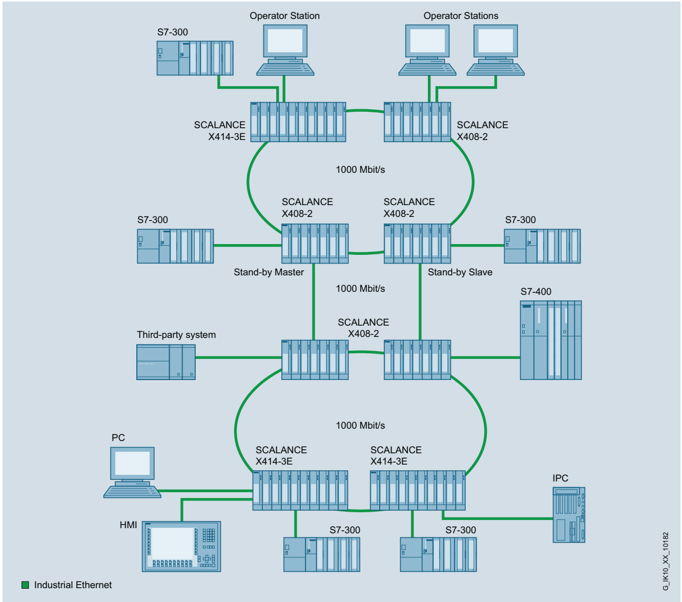
Acoplamiento redundante óptico de dos subredes Gigabit ópticas con SCALANCE X408-2 en el nivel Layer 2 y 3
