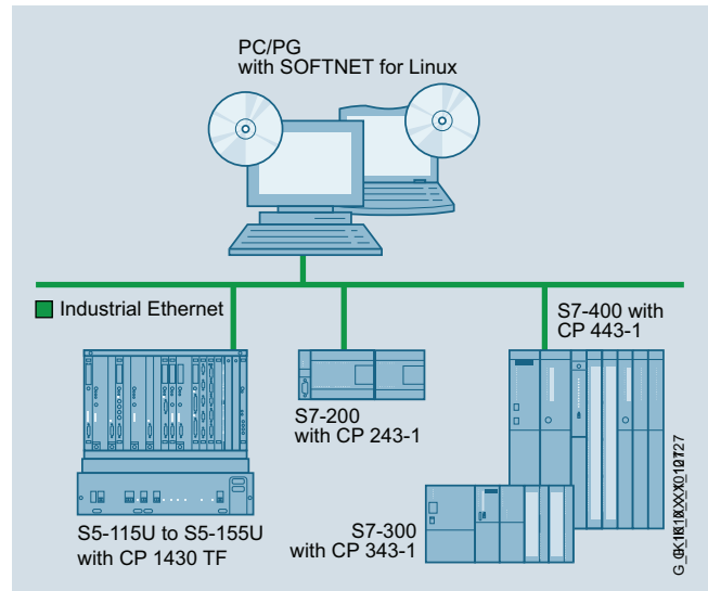
Configuración del sistema SOFTNET-S7/Linux
