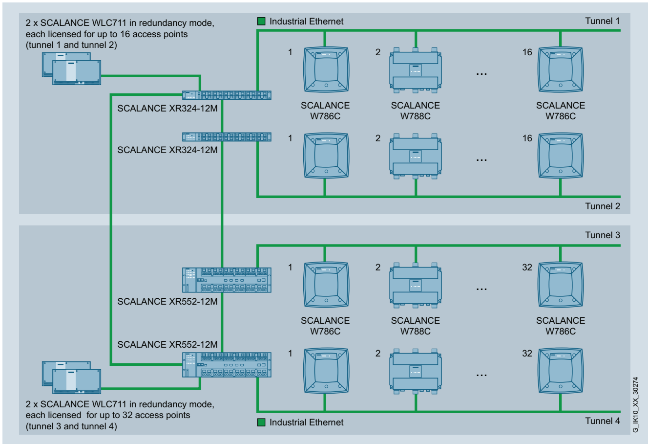
Controlador IWLAN SCALANCE WLC711 en funcionamiento redundante
