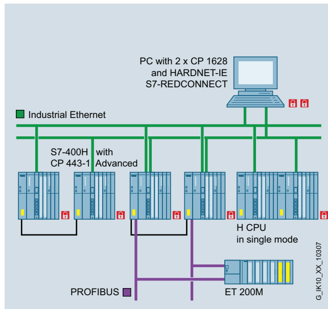
Ejemplo de construcción de red redundante y segura con CP 1628 y HARDNET-IE S7-REDCONNECT
