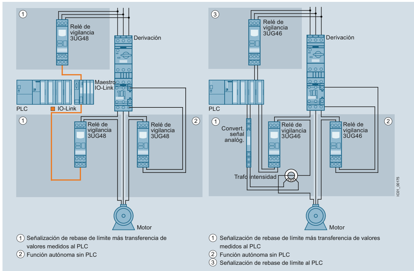
Posibilidades de la conexión de relés de vigilancia a IO-Link o de forma convencional
