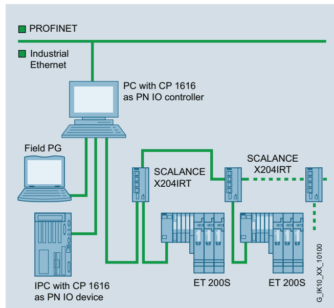
Ejemplo de configuración con SCALANCE X204IRT
