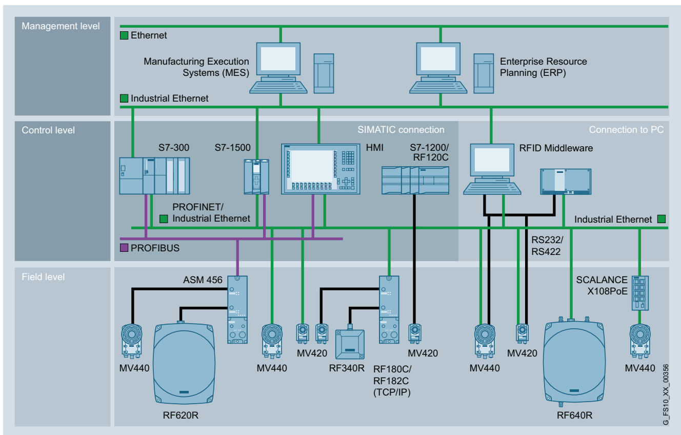
Integración de RFID en la red PROFINET/Ethernet
