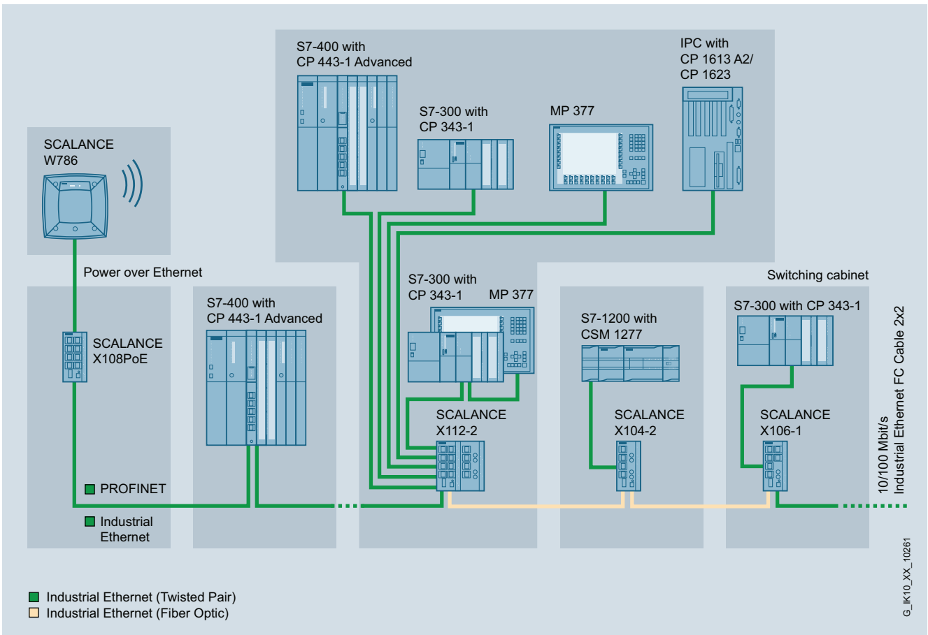
Red eléctrica y óptica con topología en línea con SCALANCE X112-2, X104-2 y X106-1, así como integración y alimentación de terminales con Power-over-Ethernet (PoE) vía SCALANCE X108PoE
