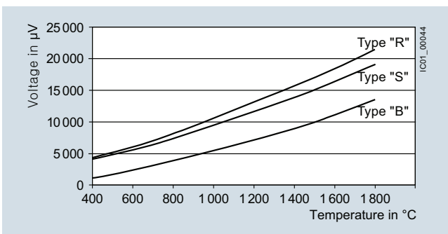
Características para sensores de tipo S, R y B
