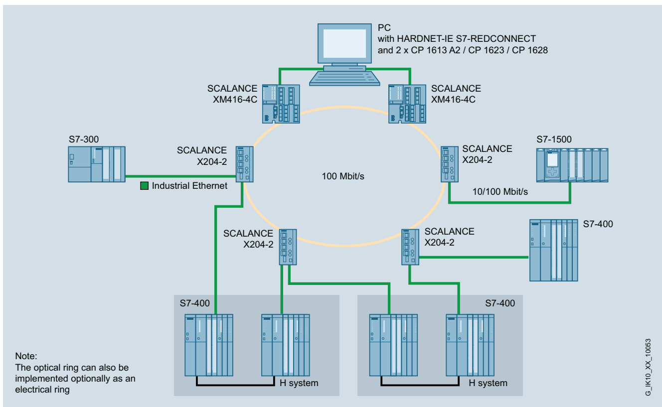
Anillo óptico redundante para conectar sistemas de alta disponibilidad
