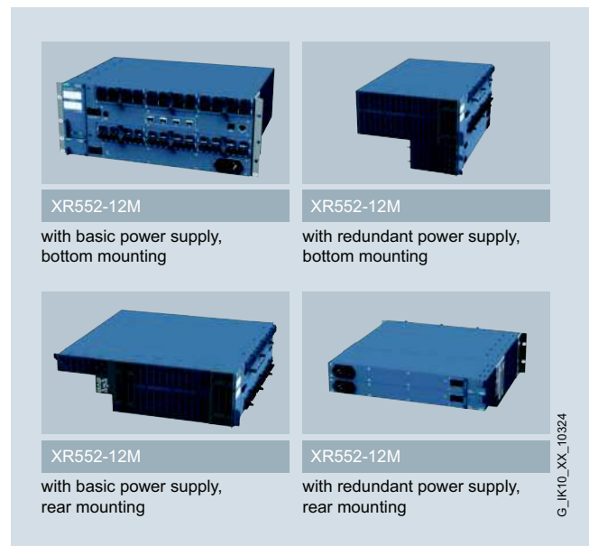
Posibilidades de montaje de una fuente de alimentación sencilla/redundante en SCALANCE XR552-12M
