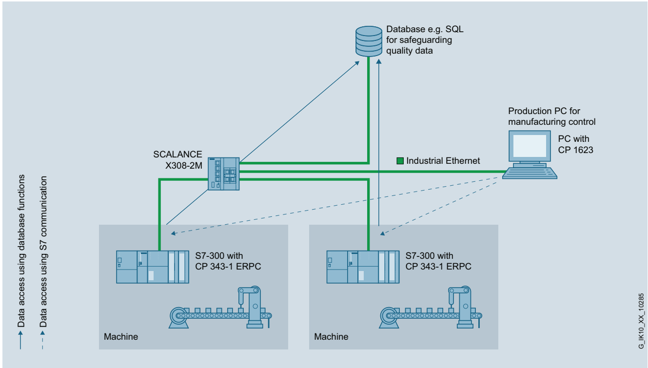
Ejemplo de configuración para archivar datos de calidad con CP 343-1 ERPC
