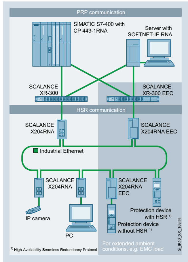
Transición redundante de una topología de red HSR en anillo a una topología PRP paralela por medio de SCALANCE X204RNA
