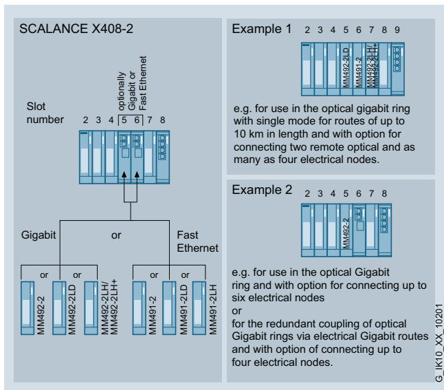
Posibilidades de aplicación de los módulos de medio con SCALANCE X408-2
