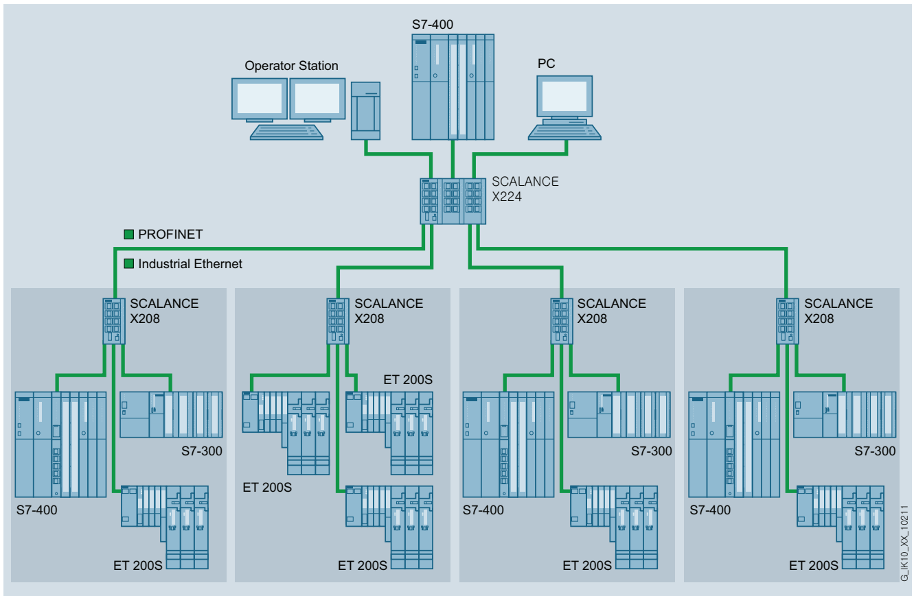
Red con topología en estrella con SCALANCE X224
