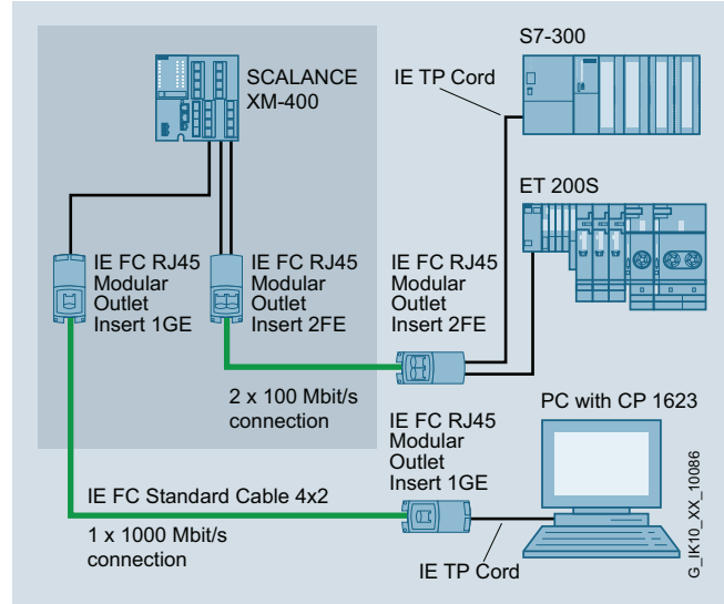
Configuración del sistema con IE FC RJ45 Modular Outlet 100 Mbit/s y 1000 Mbit/s
