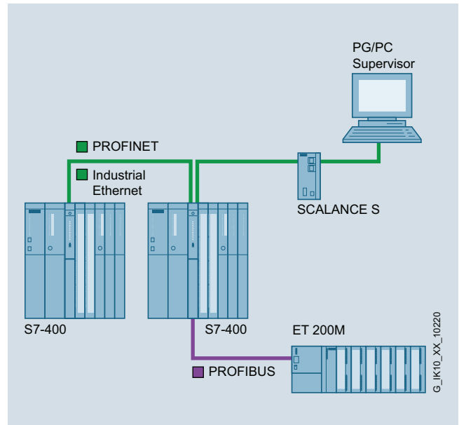
Topología en línea a nivel de gestión con switch integrado de 2 puertos
