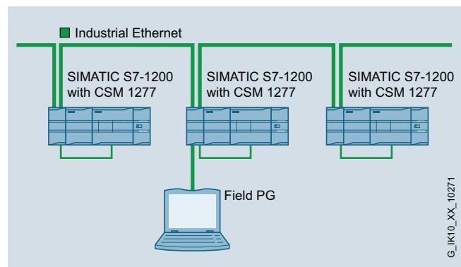
Topología en línea con CSM 1277
