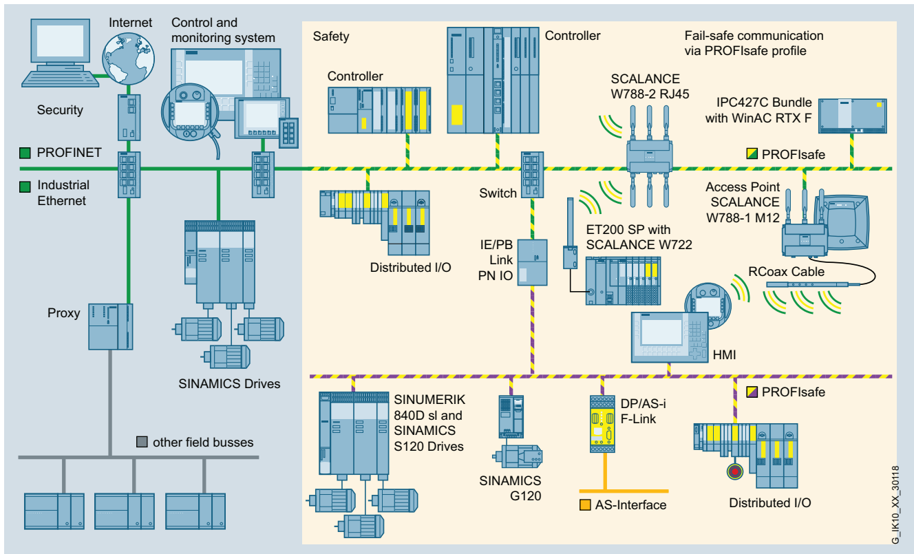
Comunicación inalámbrica de seguridad con PROFI-safe
