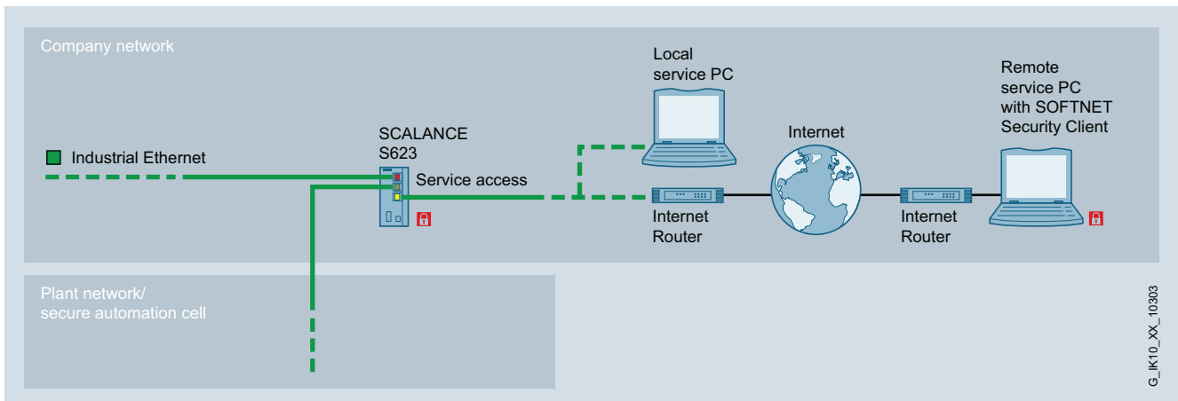
Conexión de un PC de servicio local o remoto (con acceso a Internet) a través del puerto DMZ del SCALANCE S623
