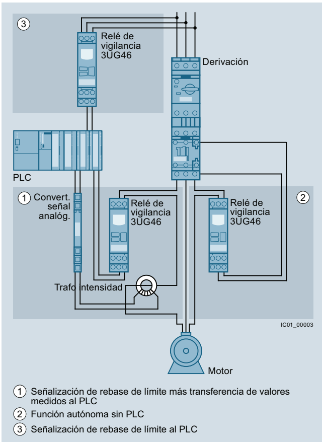
Utilización de relés de vigilancia convencionales
