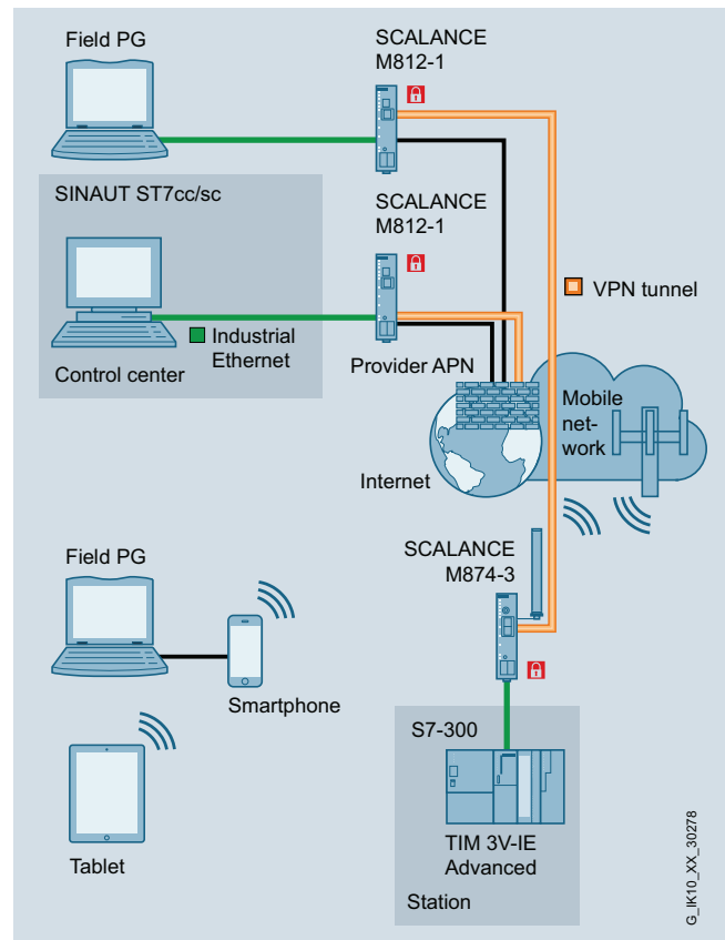
Acceso remoto a través de una conexión a Internet basada en UMTS
