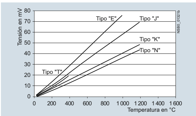
Características para sensores de tipo K, N, J, E y T
