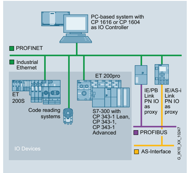
Conexión a red de nivel superior y sistema basado en PC
