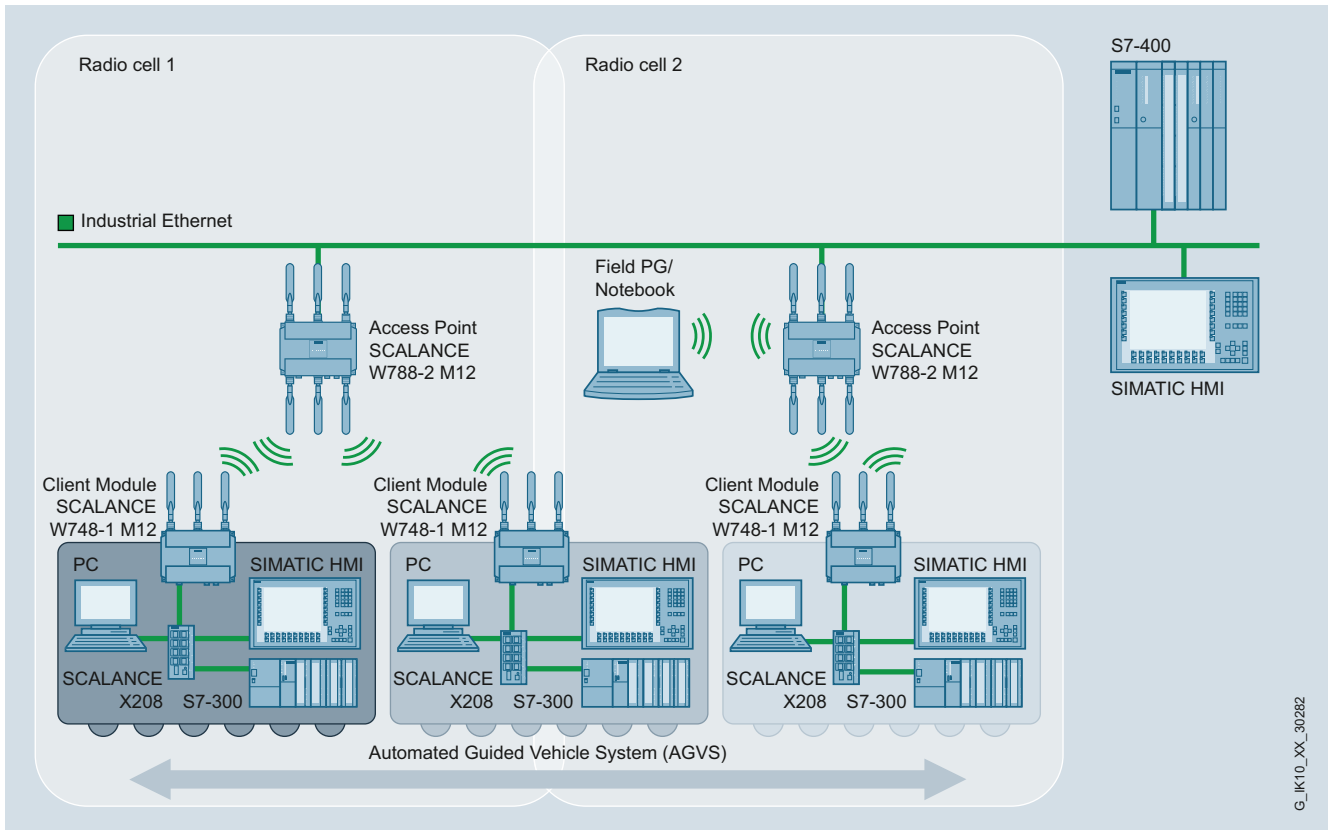
Itinerancia de equipos móviles (p. ej. Field PG y PLC móvil) en una red inalámbrica con dos puntos de acceso
