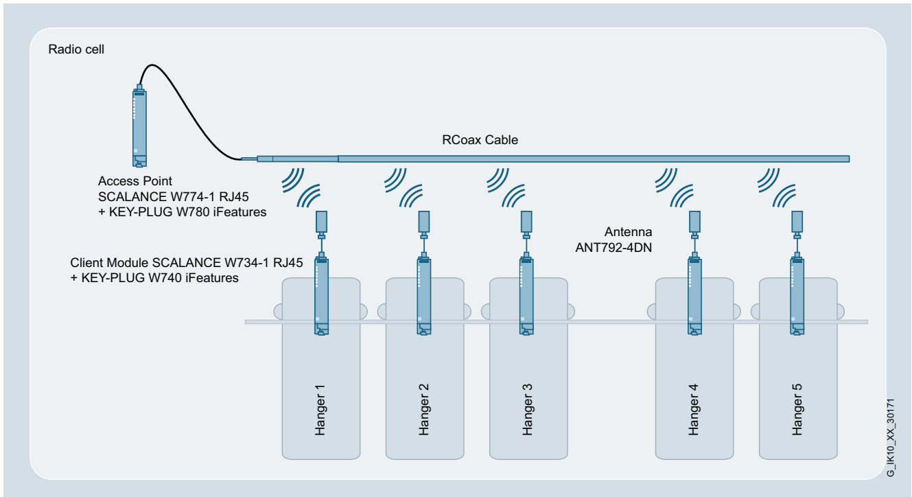
Integración de un sistema de transporte filoguiado mediante iPCF con SCALANCE W774-1 RJ45 y KEY-PLUG W780 iFeatures
