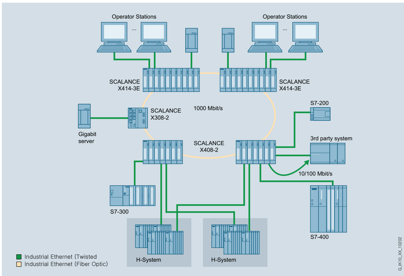
Sistema de alta disponibilidad con SCALANCE X-400
