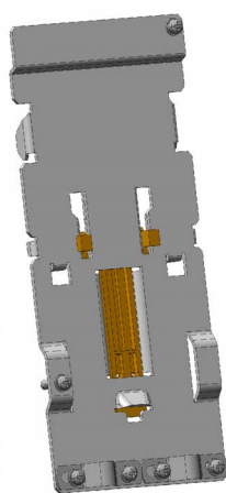
Juego de perfil DIN para tamaño de bastidor A
