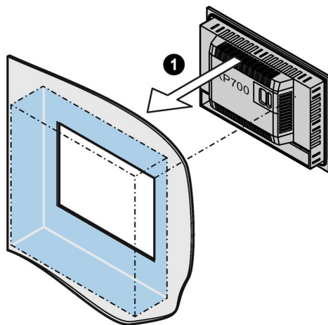
Clips de montaje para variantes de 4":
