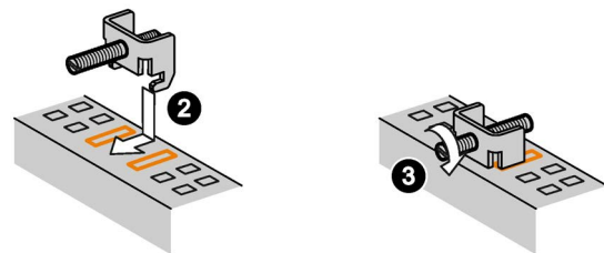
Clips de montaje para variantes de 15", 19" y 22":
