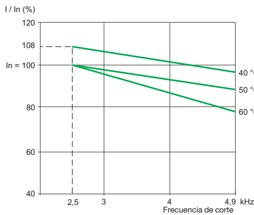
ATV 61HC25Y
