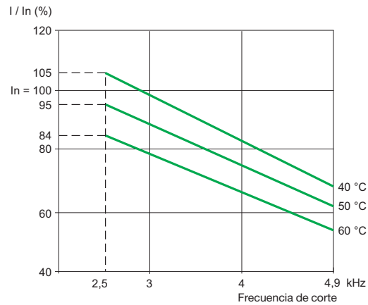
ATV 61HC20Y
