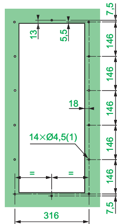
Corte y taladro
