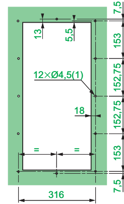
Corte y taladro
