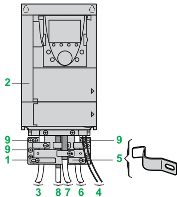
ATV 61H075N4...HD18N4
