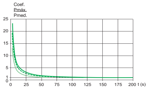
VW3 A7 805 (P permanente = 44 kW)
