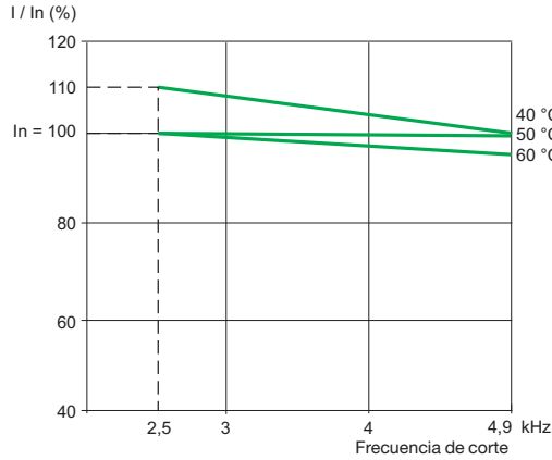
ATV 61HC11Y
