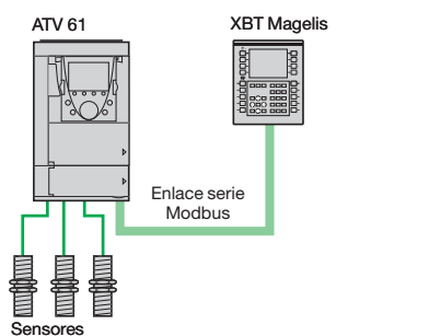
Máquina independiente con cableado hilo a hilo
