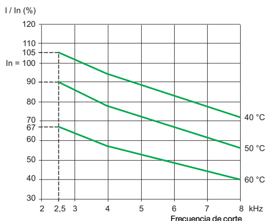
ATV 61HC22N4 asociado a un motor de 220 kW
