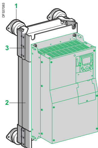
Variador ATV 61HD45N4 montado en DNV VW3 A9 628
