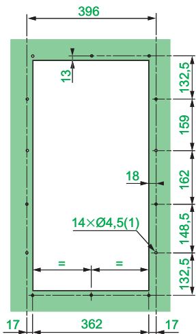
Corte y taladro
