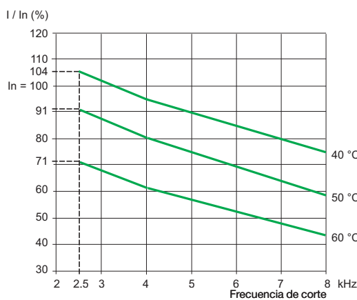
ATV 61HC31N4 asociado a un motor de 315 kW
