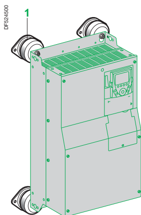
Variador ATV 61H...Y montado en kit DNV VW3 A9 643
