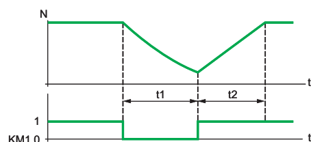
Ejemplo de corte del contactor de salida
