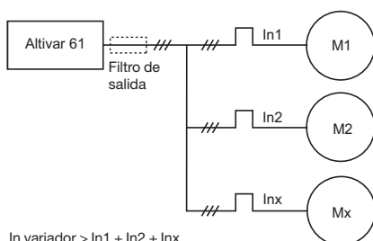
Asociación de motores en paralelo
