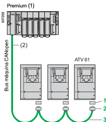
Ejemplo de esquema CANopen
