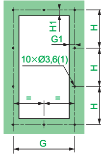
Corte y taladro
