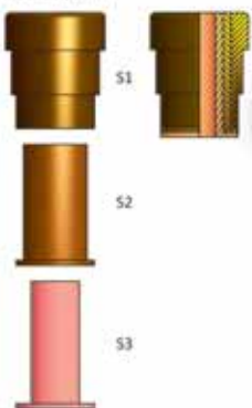
Detalle junta
