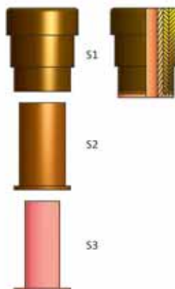
Detalle junta
